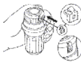
2) Paigaldage vargusevastane klamber oma kohale, kuid ärge suruge seda lõpuni kinni
