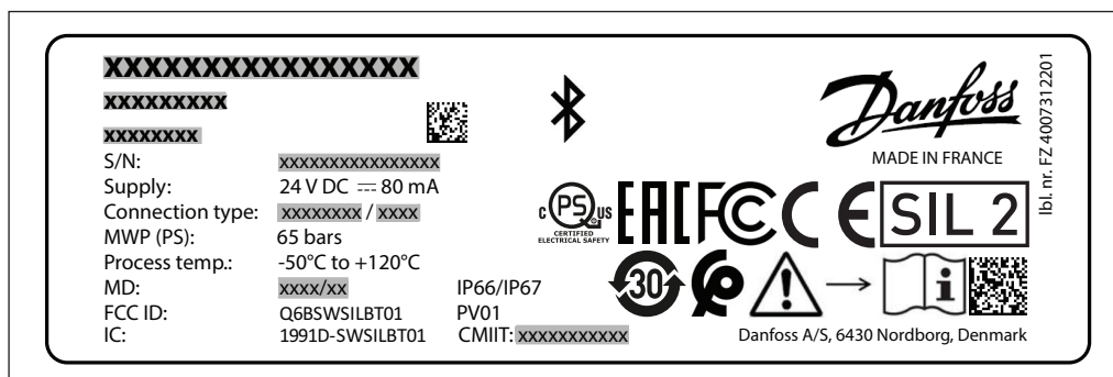
Figura 1-1: Posizione del logo SIL sulla targhetta del dispositivo sulla parte centrale destra
