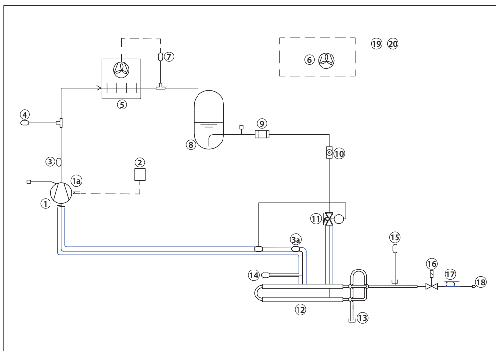
Fig. 1 - Purger R452A lay-out
