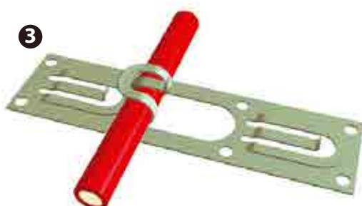
Fastgørelse af varmekablet på DEVIfast™-montagebåndet.
