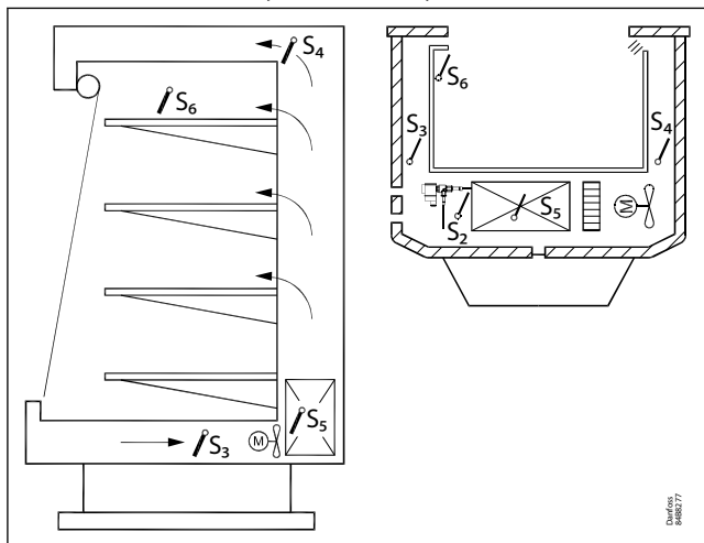
数字 22: 带一个蒸发器的背对背机柜
