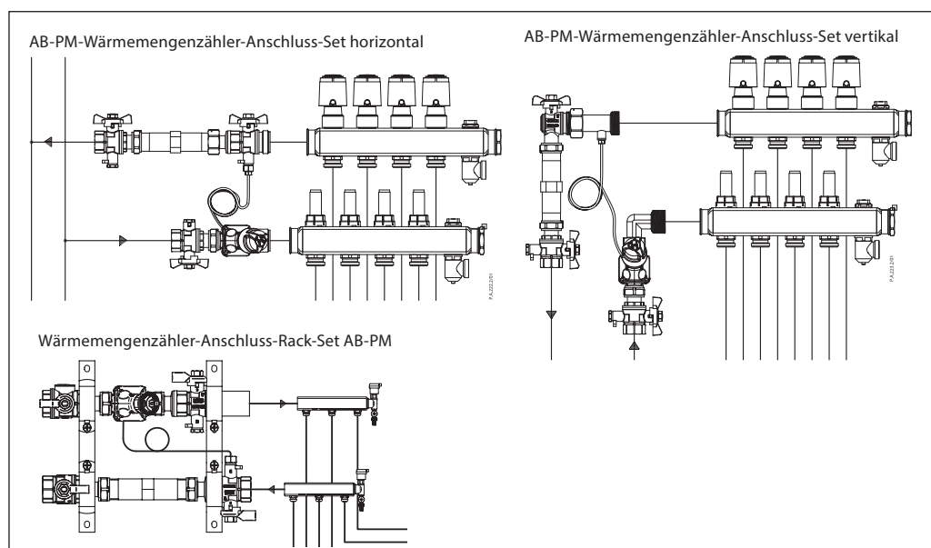
Abb. 4) AB-PM-Anschluss-Set für Verteiler (horizontaler oder vertikaler Anschluss)
