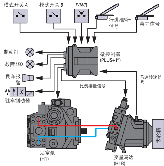
图 4：将 H1 泵与 PLUS+1 上 NFPE Control and Automotive 相结合的解决方案。
