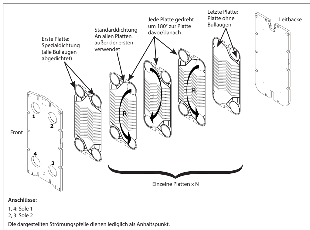
Abb. 5 Einzelne Platten: Linke und rechte Platten und Strömung
