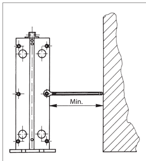
Abb. 7 Der Bereich um den Plattenwärmeübertrager muss ausreichend Platz für Wartungsarbeiten bieten
