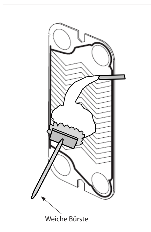
Abb. 12 Mechanische Reinigung mit weicher Bürste
