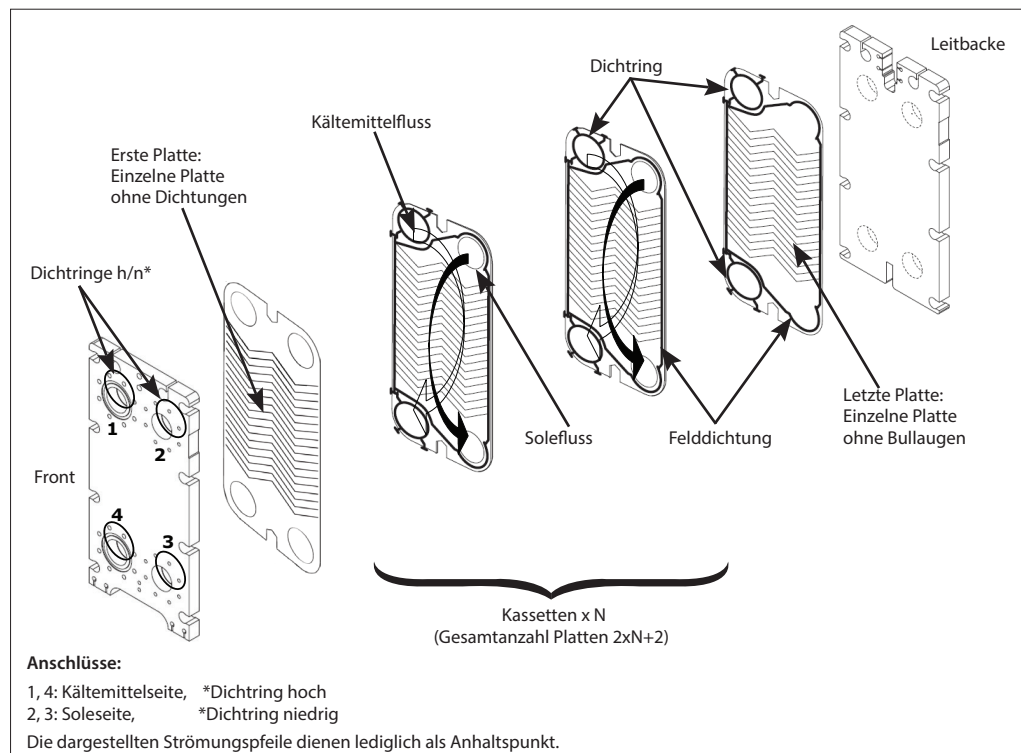
Abb. 6 Halbgewweißte Platten (Kassetten) haben keine linken oder rechten Platten. Das Kältemittel fließt stets in Port 1 und 4
