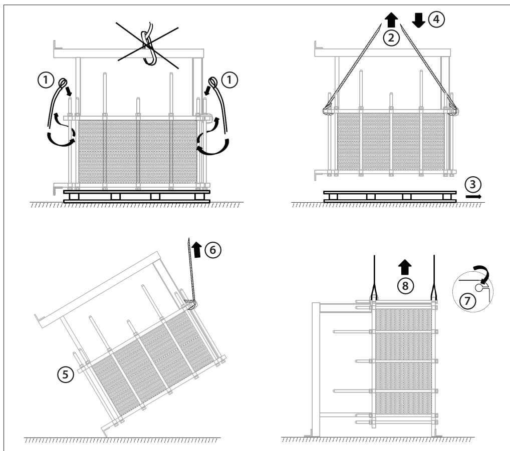
Abb. 8 Anweisungen zum Anheben
