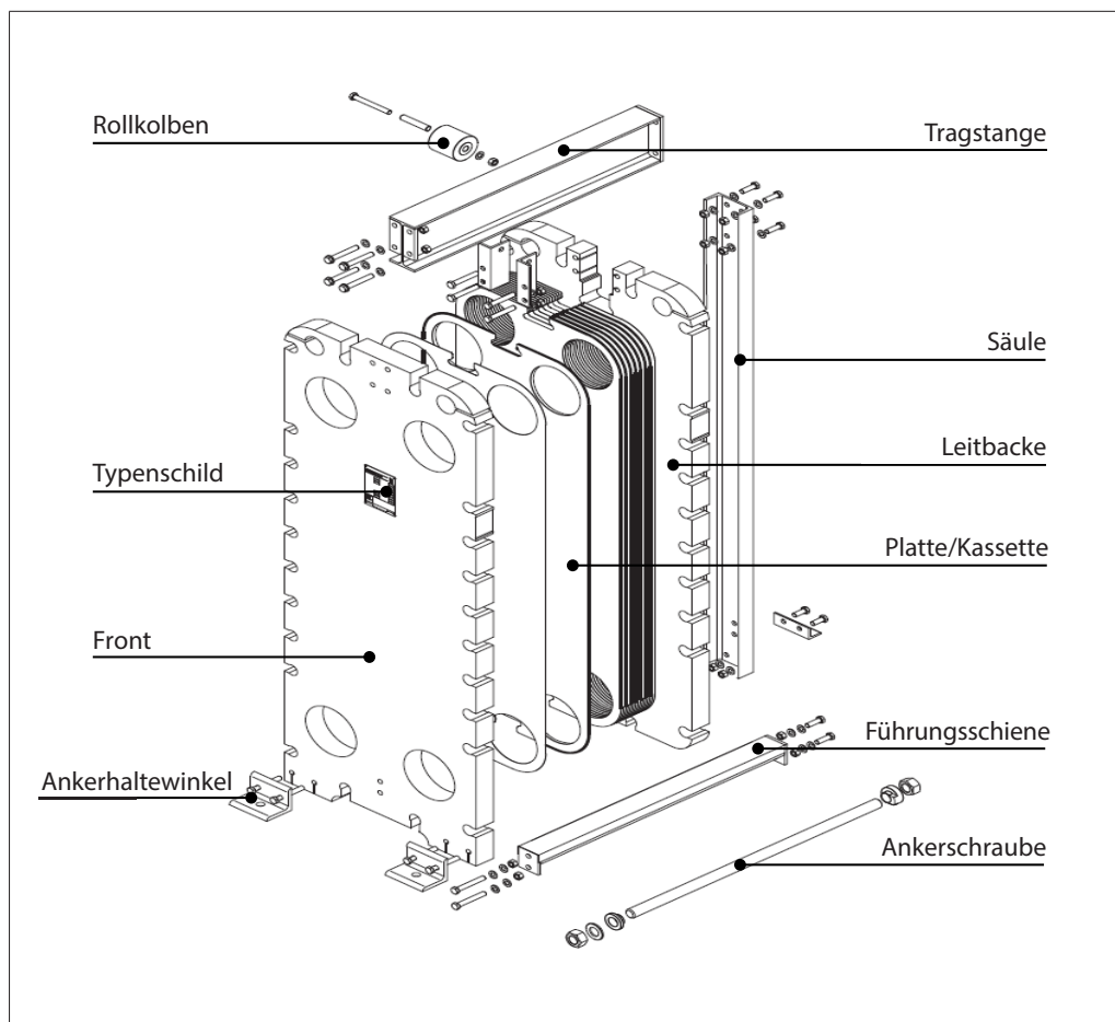
Abb. 3 Konstruktion halbggeschweißter Wärmeübertrager. Einzelplattenkonstruktion ist identisch, außer dass die Platten nicht paarweise in Kassetten (geschweißte) sind.
