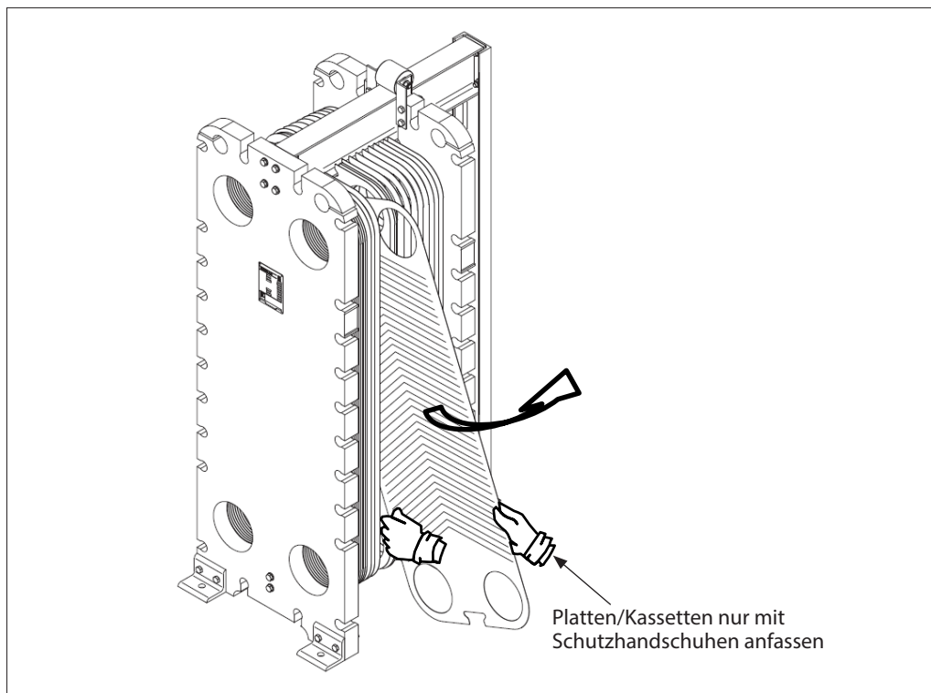
Abb. 11 Entfernen der Platten
