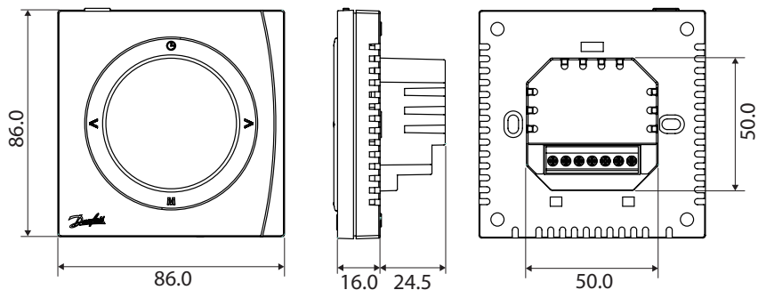
Pokojový termostat, ECtemp Next Plus
