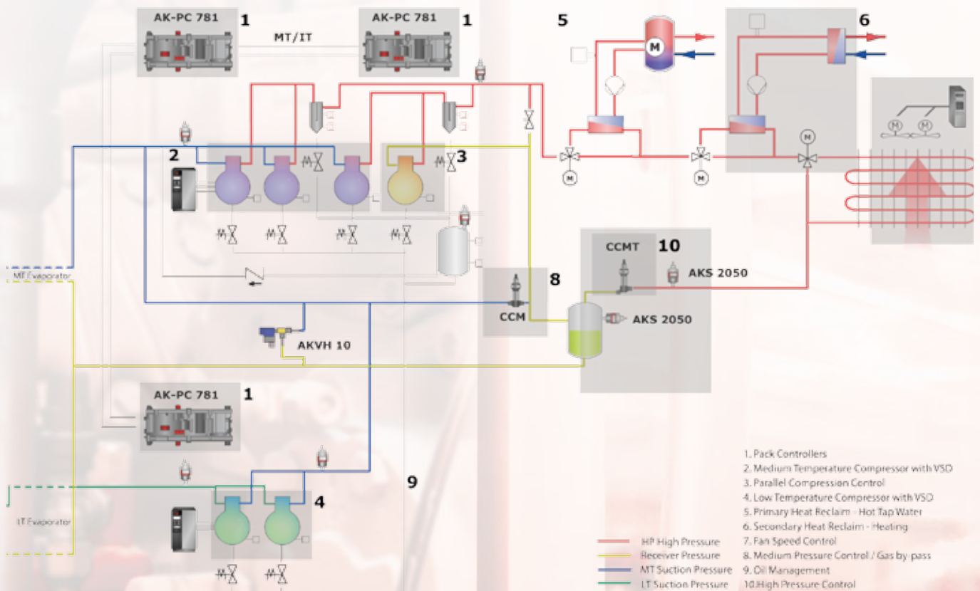
配备中间压缩机的跨临界二氧化碳增压电厂
