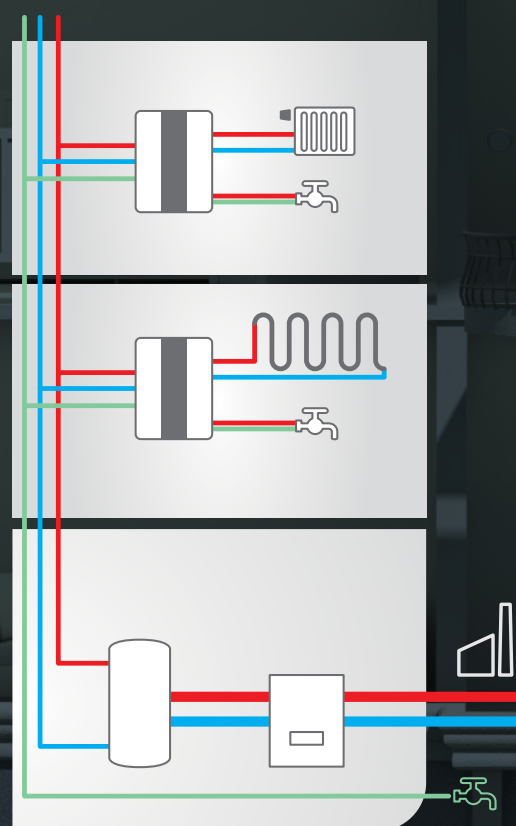
Sodobni triceveni sistem z decentralizirano distribucijo toplote in ogrevanjem sanitarne vode
