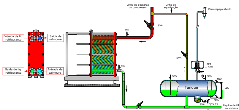
Dessuperaquecedores refrigerados a líquido (aquecimento da salmoura)
