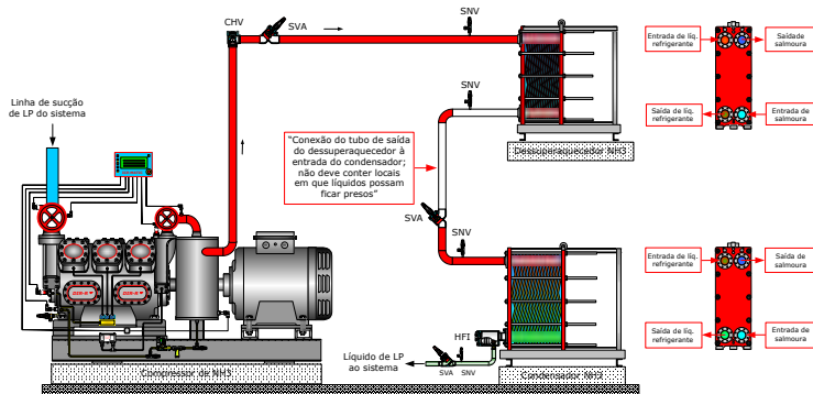
Condensadores refrigerados a líquido (aquecimento da salmoura)
