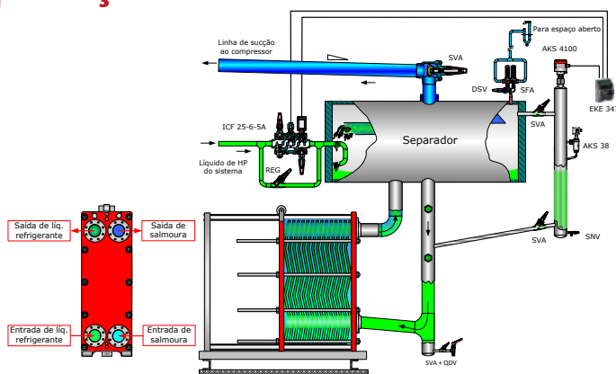
Evaporador inundado (refrigeração da salmoura)
